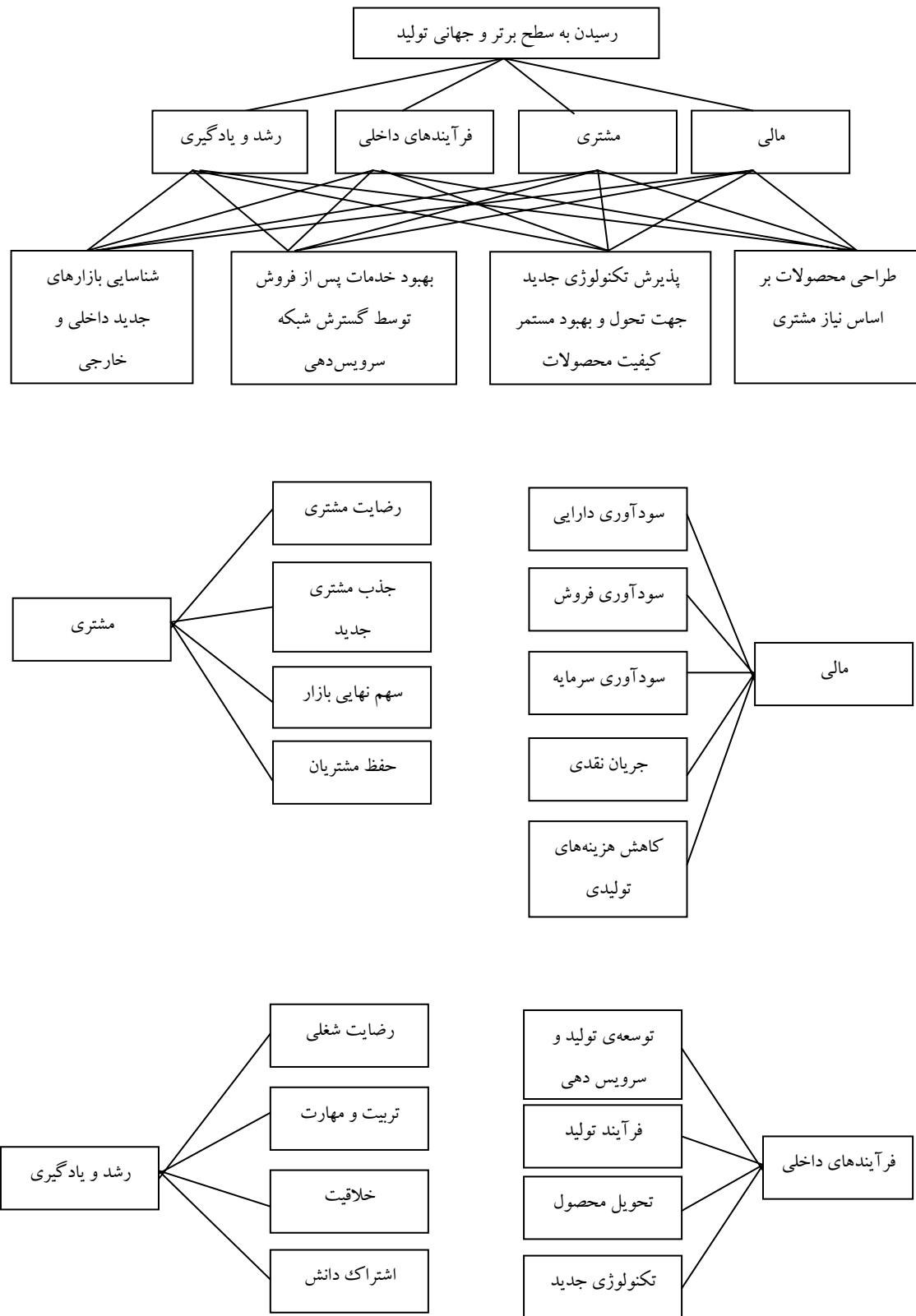
شکل ۱. ساختار سلسله مراتبی مناظر، شاخص‌ها و استراتژی‌های دستیابی به تولید کلاس جهانی
