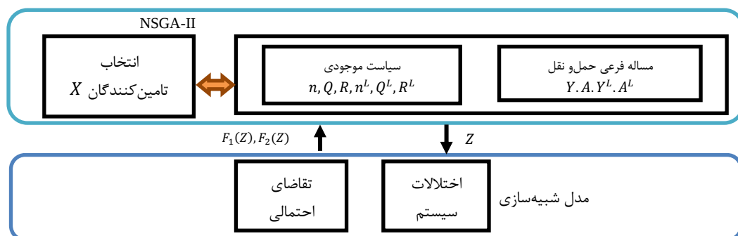
شکل ۲. نمای کلی روش بهینه‌سازی شبیه‌سازی پیشنهادی
