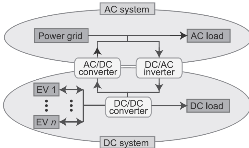
شکل ۱. شبکه برق محلی سیستم مدیریت انرژی خانگی
