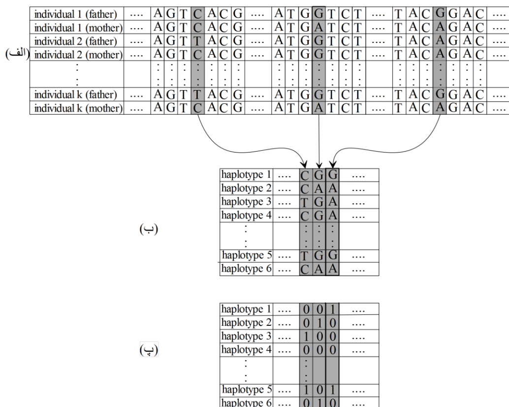
شکل ۱. الف. بخشی از کروموزوم‌های پدرانه و مادرانه در یک جمعیت نمونه. ب. هاپلوتایپ‌های متناظر کروموزوم‌ها. پ. هاپلوتایپ‌های گذشته.
