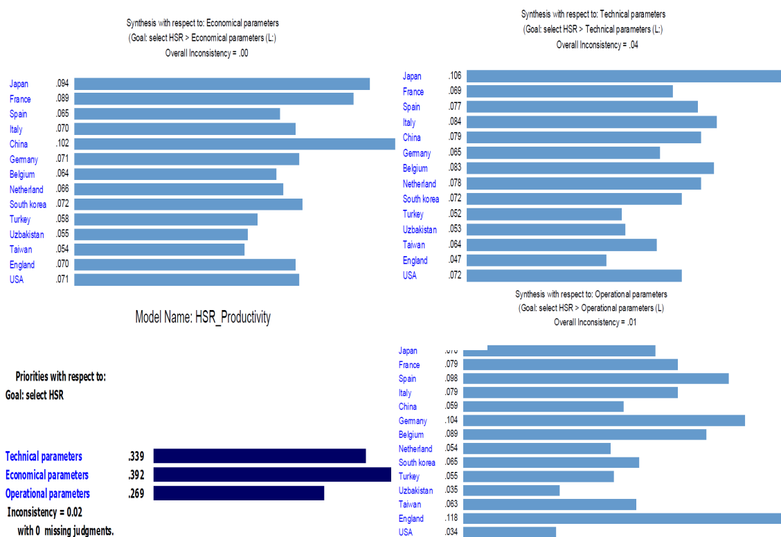
شکل ۱۳. عملکرد بهره‌وری کشورهای مختلف با توجه به (الف) پارامترهای فنی، (ب) پارامترهای اقتصادی (پ) پارامترهای بهره‌برداری و (ت) نتایج وزن دهی سه معیار اصلی
