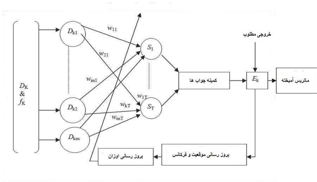
شکل ۴. الگوریتم بت
