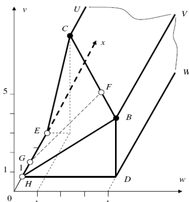
شکل ۵. مجموعه امکان تولید حاصل از تکنولوژی فار و گراسکوف با یک فاکتور انقباض
