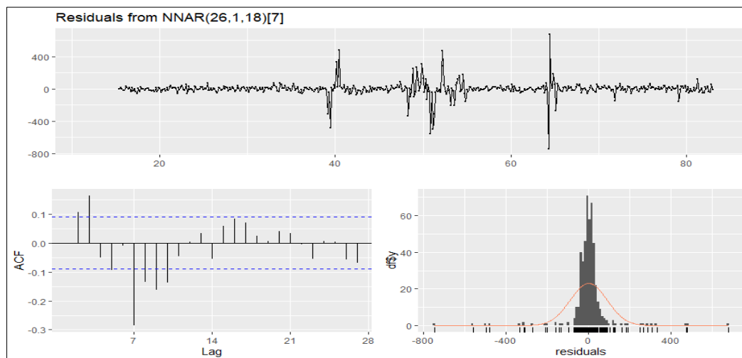
شکل ۱۶. بررسی وضعیت باقیمانده‌ها در مدل شبکه عصبی NNAR(26, 1, 18)[7] برازش یافته روی داده‌های تمام روزهای هفته
