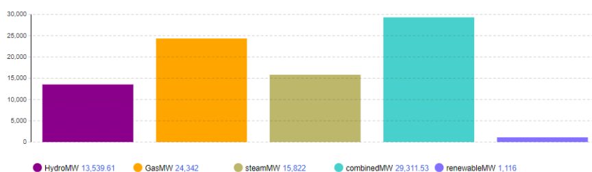
شکل ۳. ظرفیت اسمی نیروگاه‌ها در ۹۶ ماه اجرای مدل
