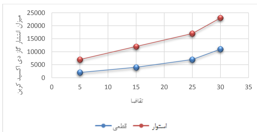
شکل ۴. مقایسه تابع هدف دوم در حالت استوار و قطعی با تغییر متغیر تقاضا
